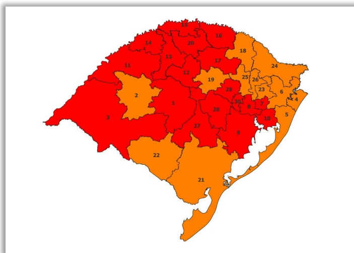
Figura 2. Regiões de saúde com incidência de casos notificados de dengue (exceto os descartados) acima do Limite Superior Endêmico (LSE) do Estado em todas as últimas quatro SE (em vermelho), acima do LSE em ao menos uma das últimas quatro SE (em laranja), regiões que estão abaixo do LSE mas possuem pelo menos um caso confirmado nas últimas quatro SE (em amarelo), regiões que estão abaixo da LSE e que não possuem caso confirmado nas últimas quatro SE (em branco), RS, 2023*
