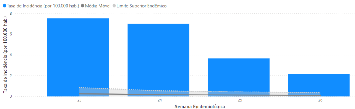
Figura 1. Taxa de Incidência de casos notificados exceto descartados de dengue no RS, SE 23 a 26/2023*
