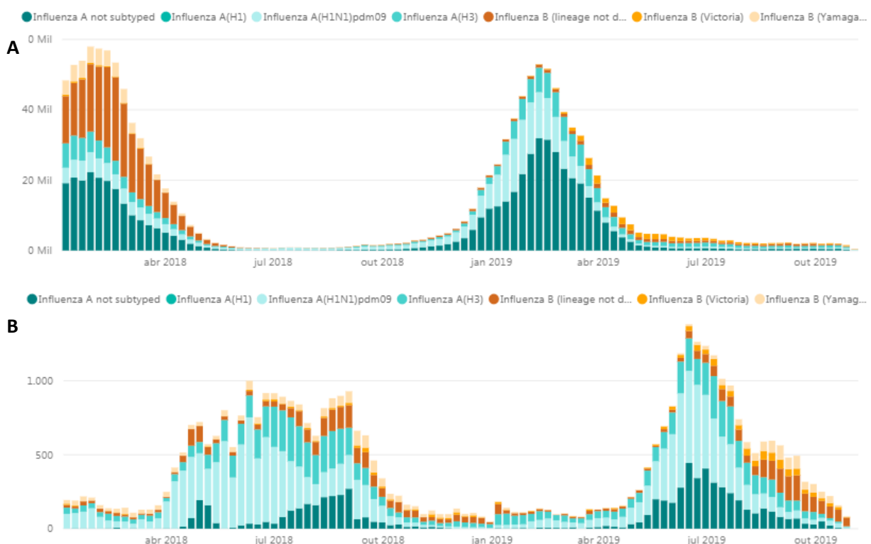
Figura 1 Histograma comparativo da circulação de Influenza no mundo (1A) com América do Sul (1B) no período de 2018 a 27/10/2019
